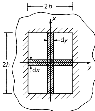
Fig. 10.4. Rectangular membrane
