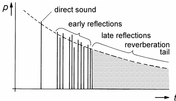
Fig. 12.10. Echogram
