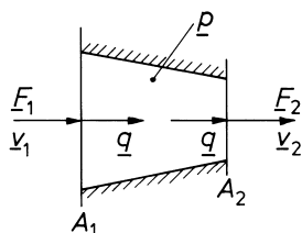
Fig. 3.4. Velocity transformer
